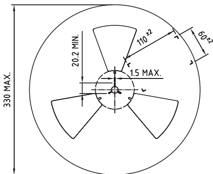
800 pcs REEL
